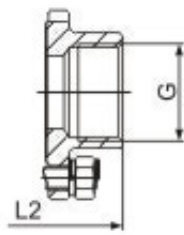
型号：GU-(16、25、 40、50)(G)
