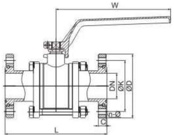
型号: GU-(16、25、40、50)(F)
